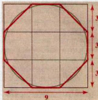
Современный чертёж
